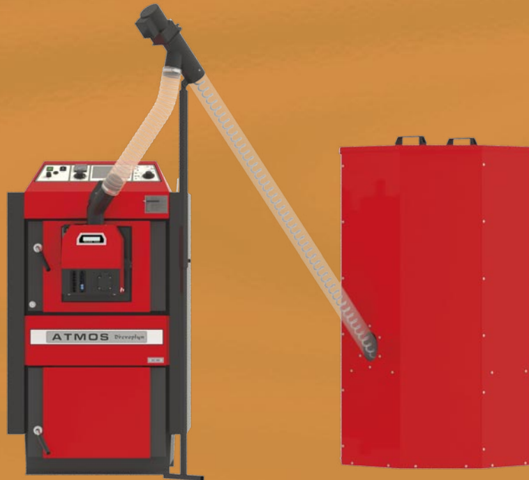
Standardowe zestawienie Kocioł DC 25 PSX z podajnikiem DA2000 – 2 m oraz zasobnikiem 500 l (1000 l) Całkowita szerokość zestawu około 2020 mm (2300)
